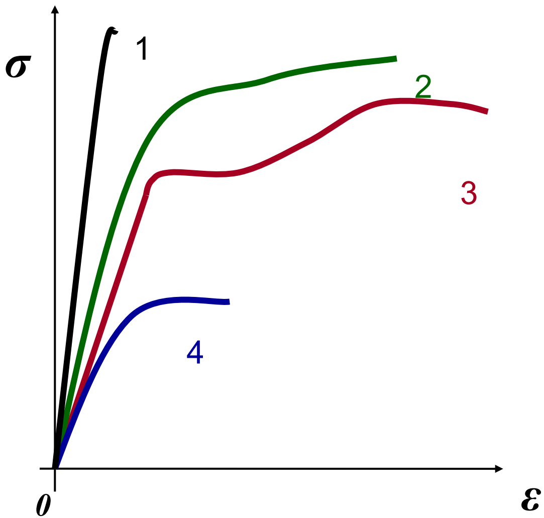
26. Диаграмма растяжения малоуглеродистой стали 3: 1); 2); 3); 4).
